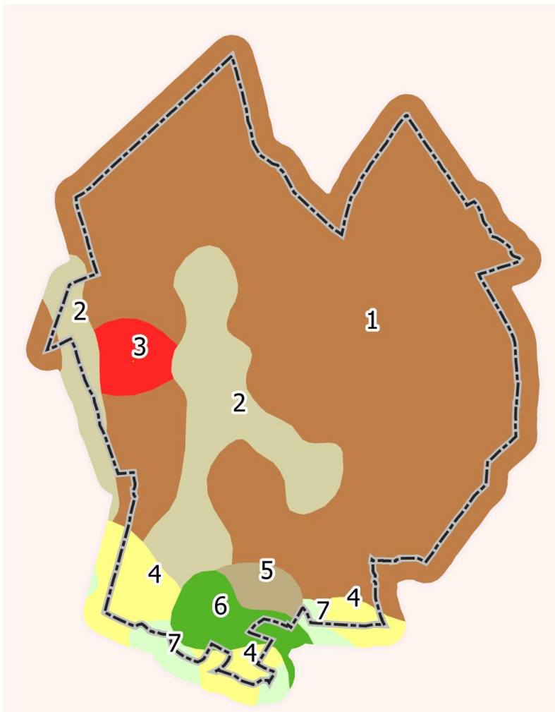
Mapa. Mapa utworów powierzchniowych – zrzut z Mapy Geologicznej Polski wykonanej w skali 1:500 000 (warstwa źródłowa: https://dane.gov.pl/pl/dataset/772,mapa-geologiczna-polski-w-skali-1500-000/resource/30465/table )
